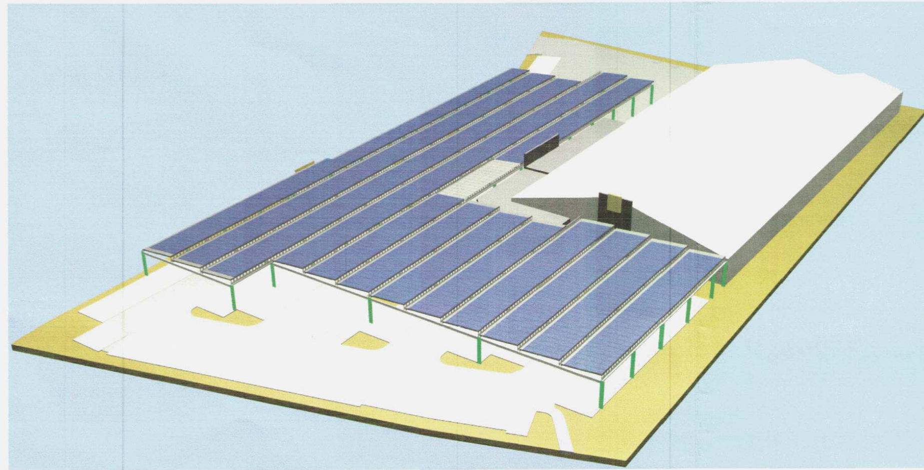
Ansicht von Süd-Osten
