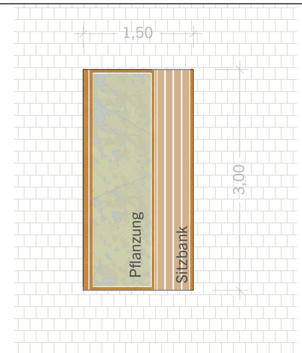
Pflanzkübel, Grundriss
