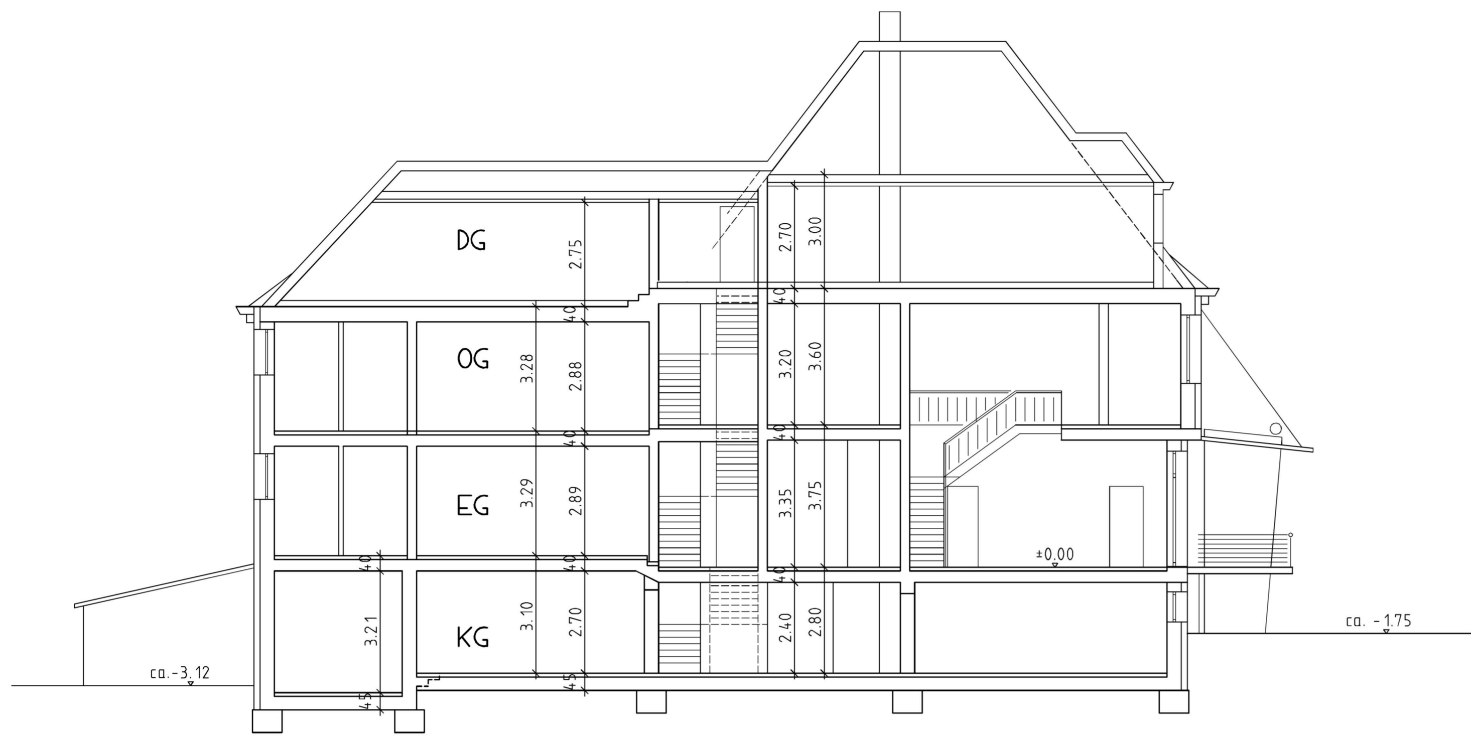
SCHEMASCHNITT
