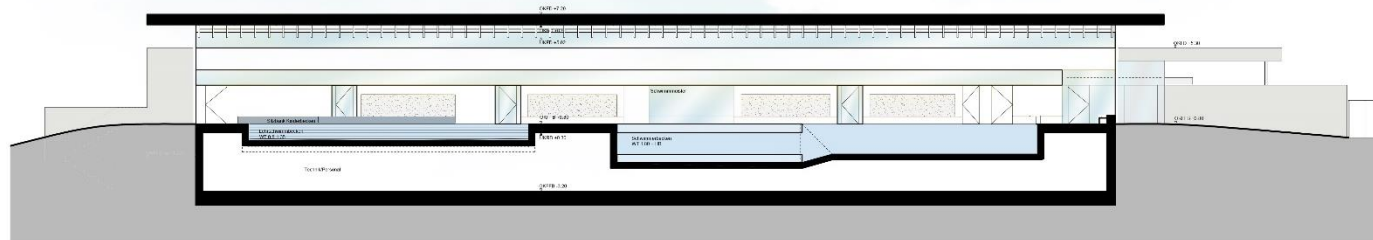
Schnitt CC – mit Hubboden W.T. 1,80m
