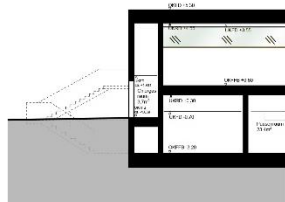
Schnitt BB
