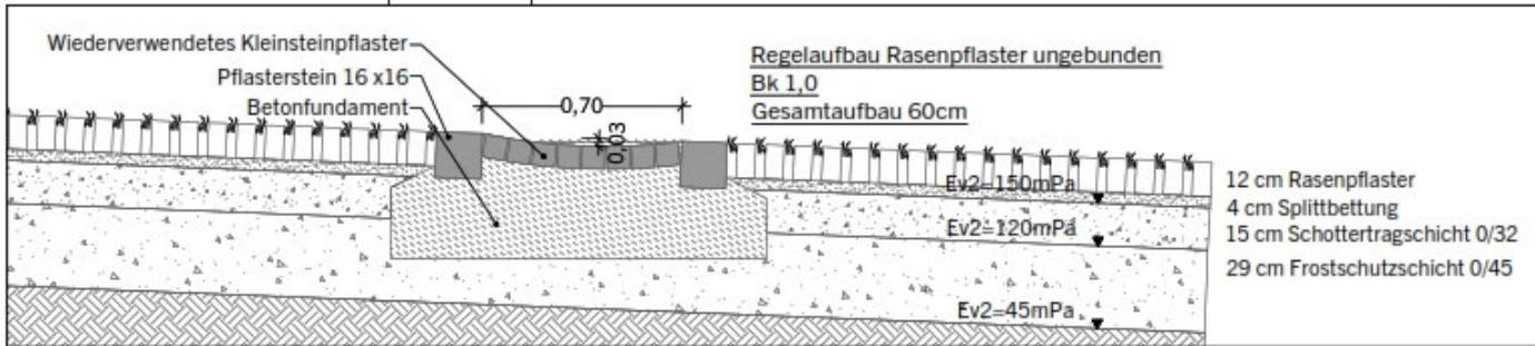
Prinzipanschnitt Wasserlauf in Rasen
