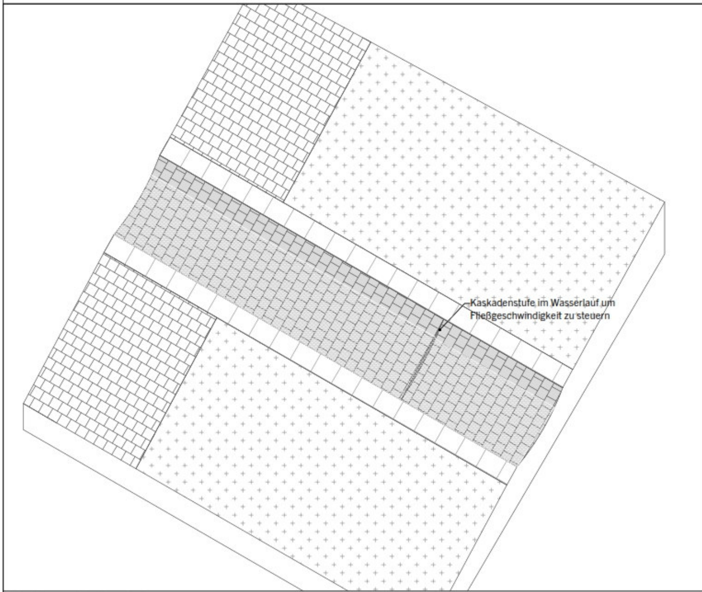
Prinzip-Axonometrie Wasserlauf
