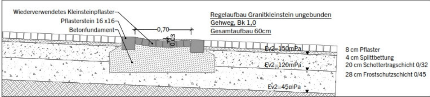
Prinzipanschnitt Wasserlauf in Gehweg
