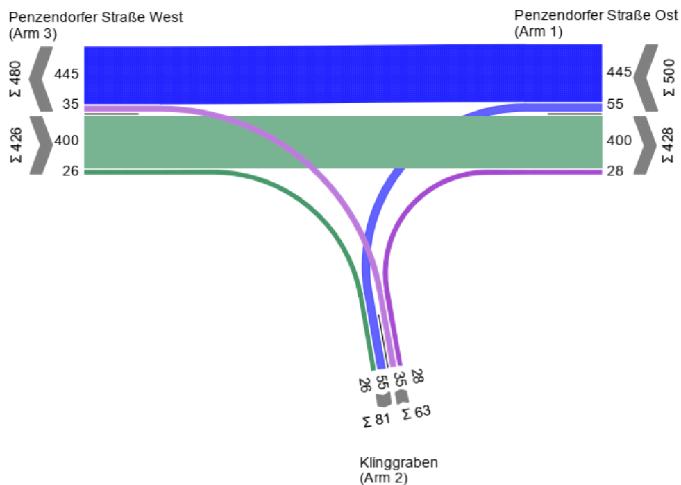
Anhang 104: KP 34 Strombelastungsplan Prognosenußfall 2030, Morgenspitze
