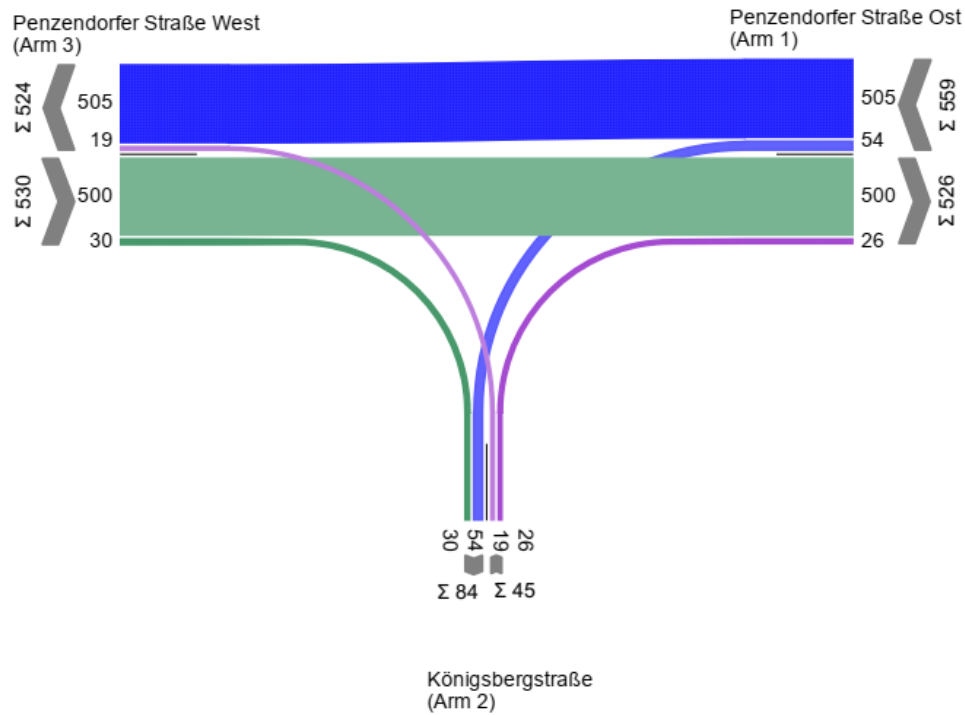
Anhang 128: KP 36 Strombelastungsplan Prognosenußfall 2030, Morgenspitze
