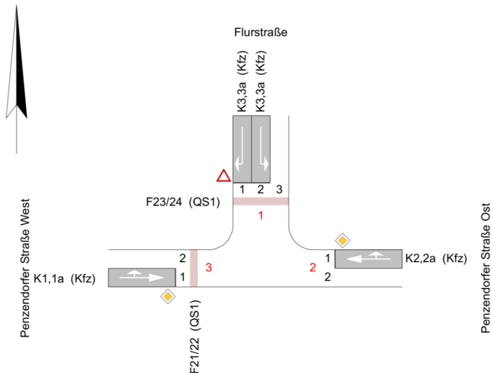
Abbildung 37: Geometrie des Knotenpunktes Penzendorfer Straße/Flurstraße mit Kennzeichnung der Nomenklatur (Quelle: LISA6.2.0)
