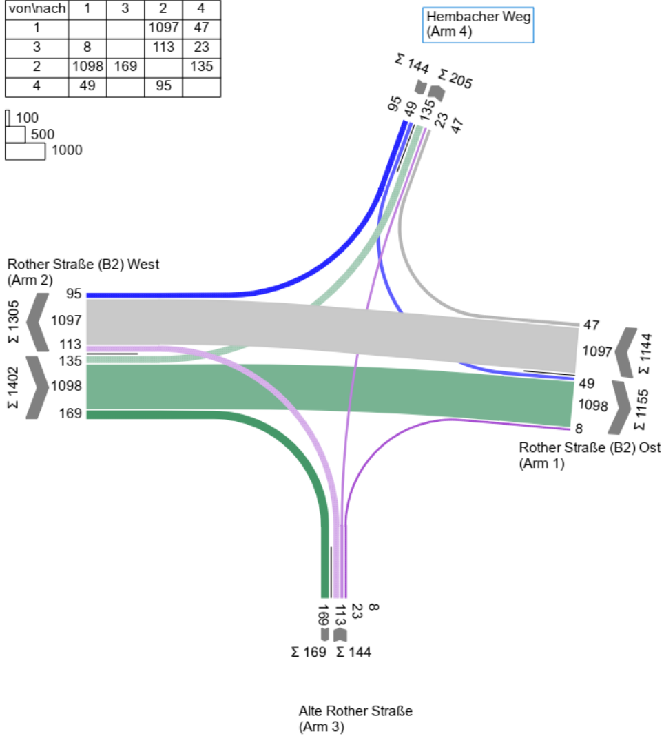
Anhang 81: KP 32 Strombelastungsplan Prognosenußfall 2030, Abendspitze
