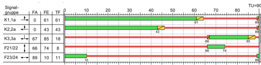
Abbildung 38: Signalzeitenplan des Knotenpunktes Penzendorfer Straße/Flurstraße (Quelle: LISA6.2.0)
