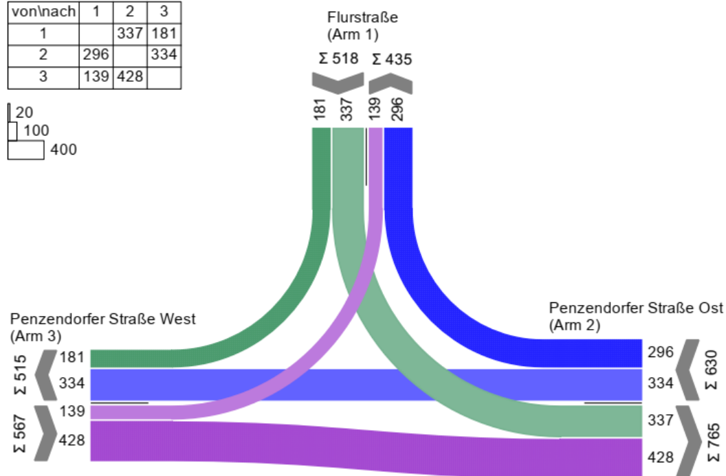
Anhang 69: KP 28 Strombelastungsplan Prognosenullfall 2030, Abendspitze
