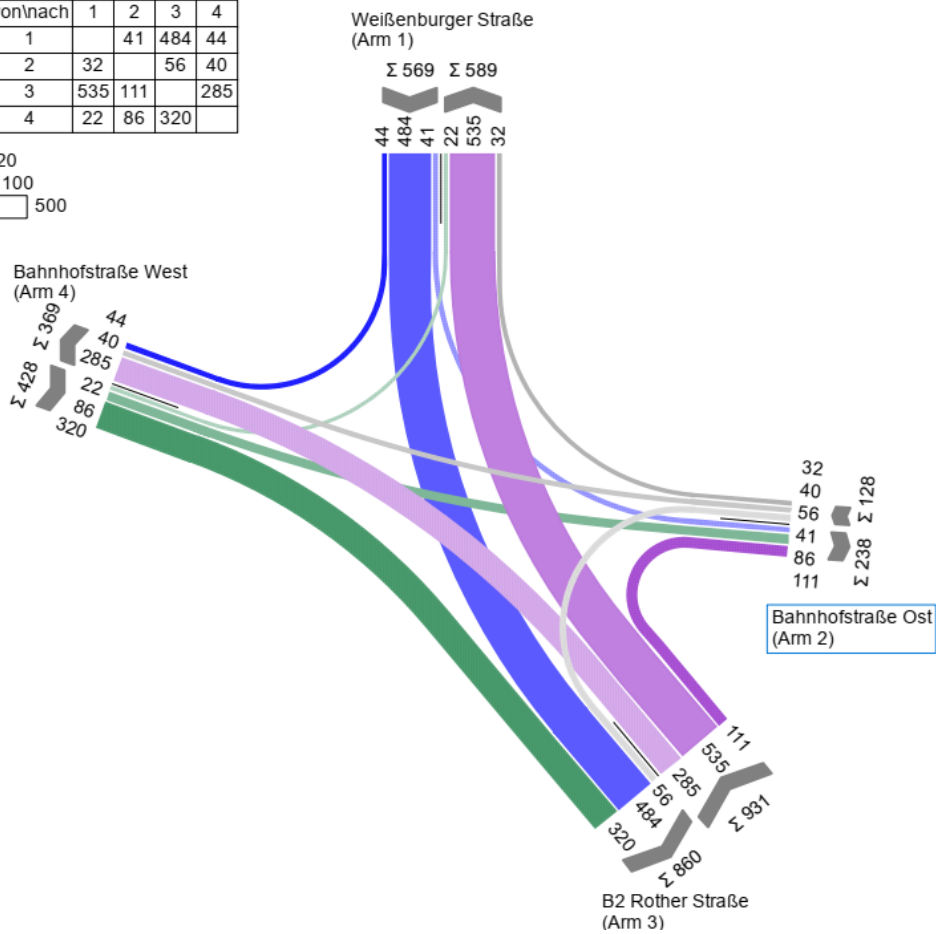
Anhang 12: KP 3 Strombelastungsplan Prognoseplanfall 2030, Morgenspitze
