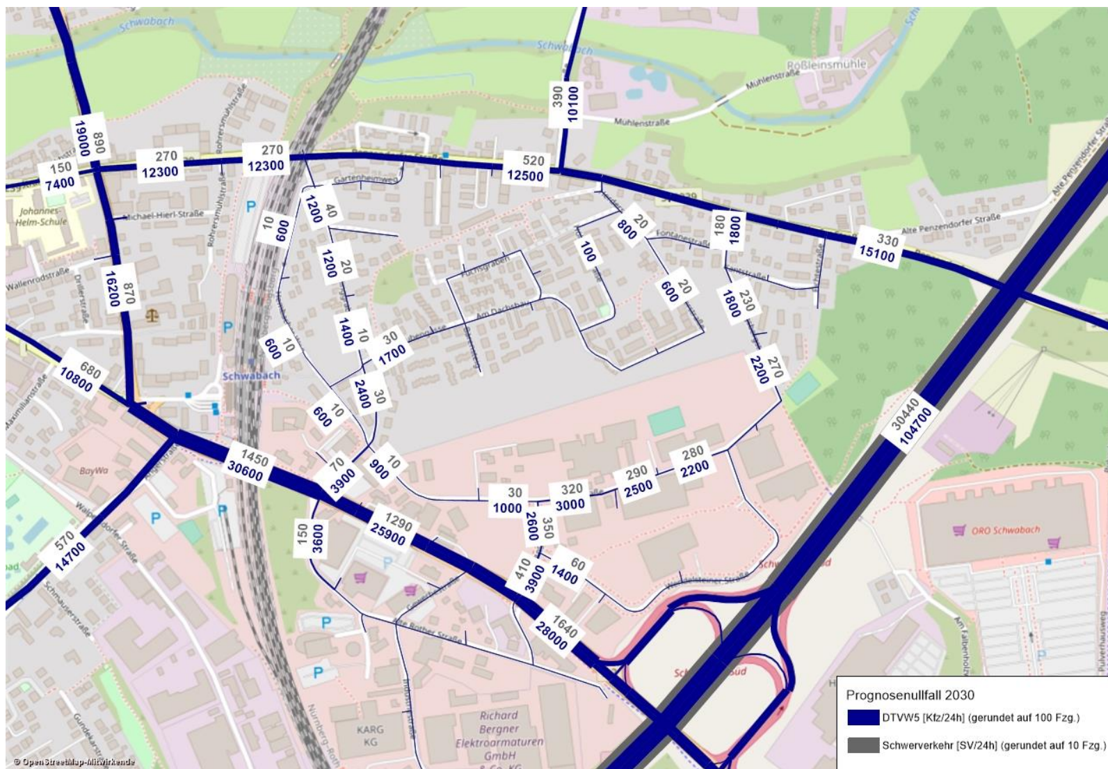
Abbildung 13: Verkehrsstärke Prognosenullfall 2030 [Kfz/24h, davon Lkw/24h] (Kartengrundlage: Open Street Map)
