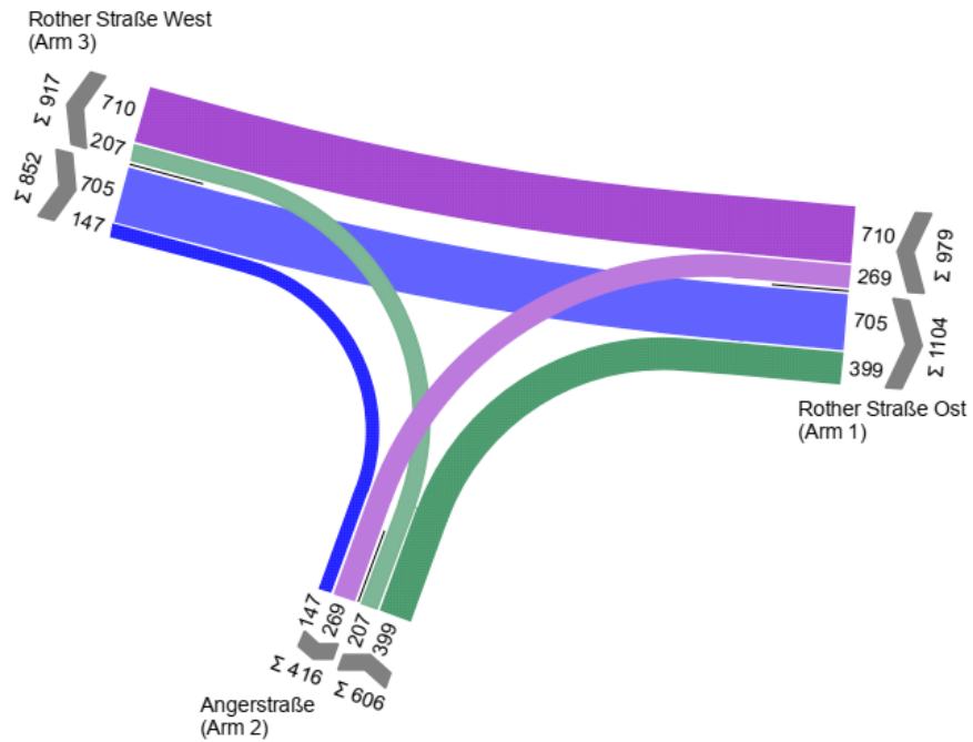
Anhang 20: KP 4 Strombelastungsplan Prognosenußfall 2030, Morgenspitze
