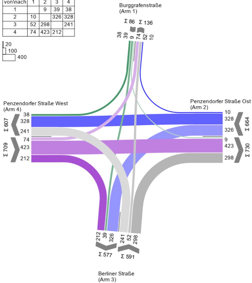
Anhang 57: KP 27 Strombelastungsplan Prognosenullfall 2030, Abendspitze
