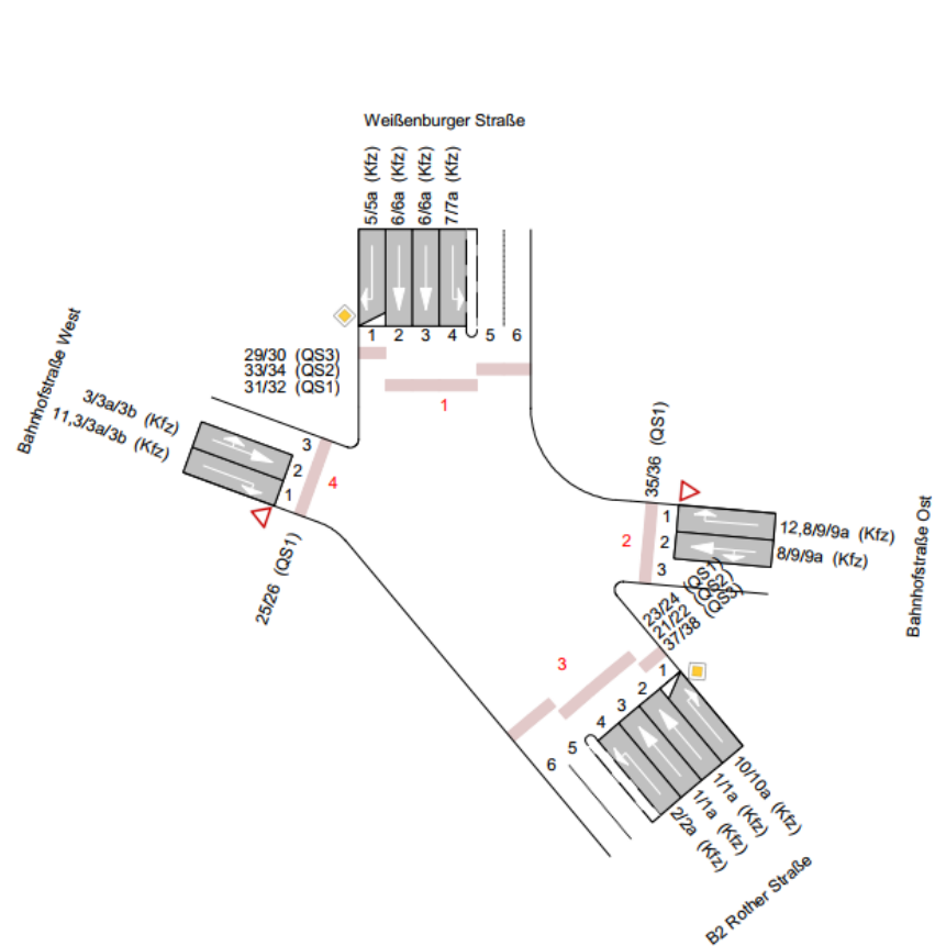
Abbildung 26: Geometrie des Knotenpunktes Bahnhofstraße/Weissenburger Str./Rother Straße mit Kennzeichnung der Nomenklatur (Quelle: LISA6.2.0)
