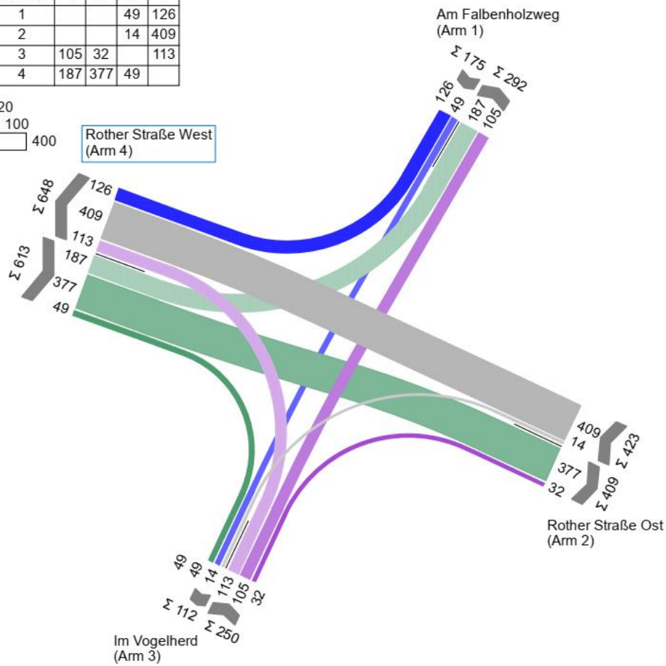
Anhang 36: KP 5 Strombelastungsplan Prognoseplanfall 2030, Morgenspitze
