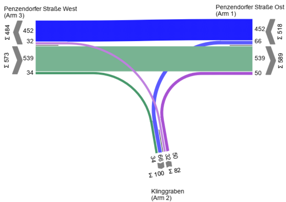
Anhang 109: KP 34 Strombelastungsplan Prognosenußfall 2030, Abendspitze
