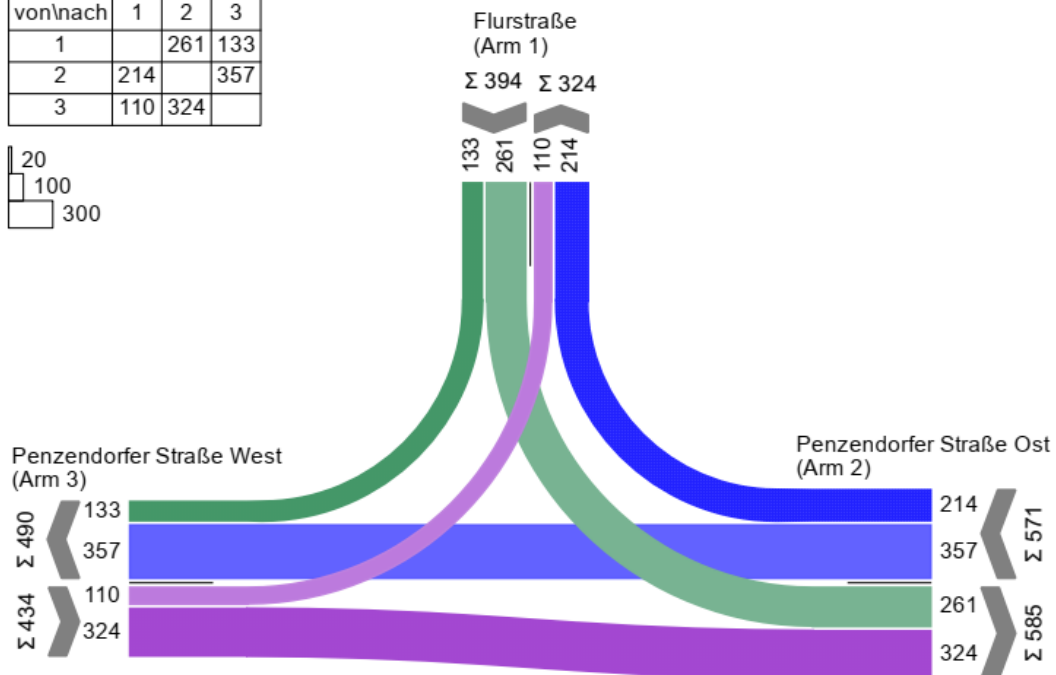
Anhang 68: KP 28 Strombelastungsplan Prognosenullfall 2030, Morgenspitze
