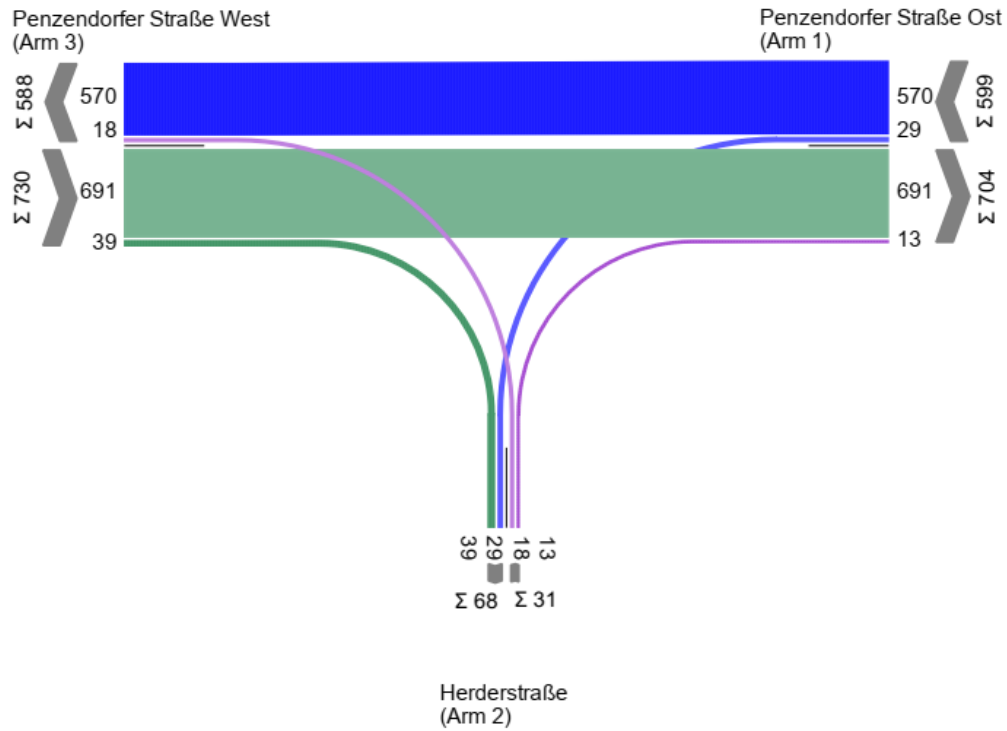
Anhang 117: KP 35 Strombelastungsplan Prognosenullfall 2030, Abendspitze
