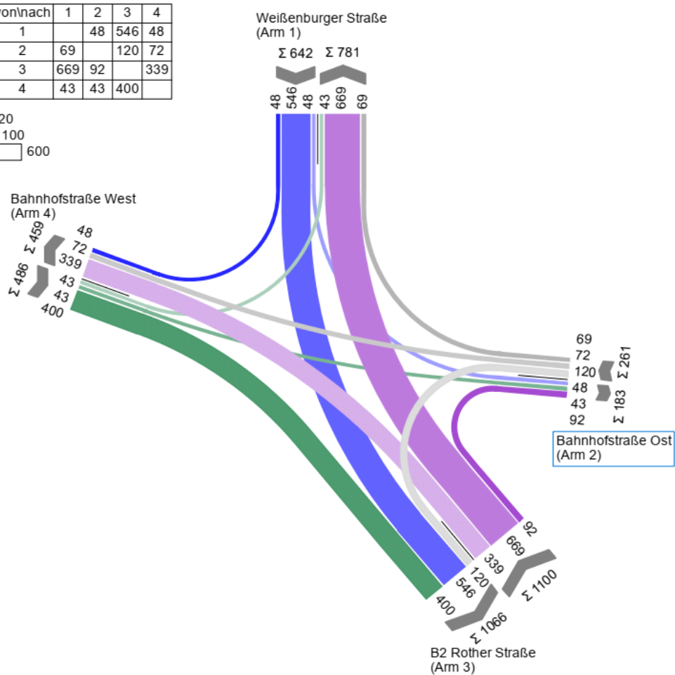
Anhang 9: KP 3 Strombelastungsplan Prognosenußfall 2030, Abendspitze
