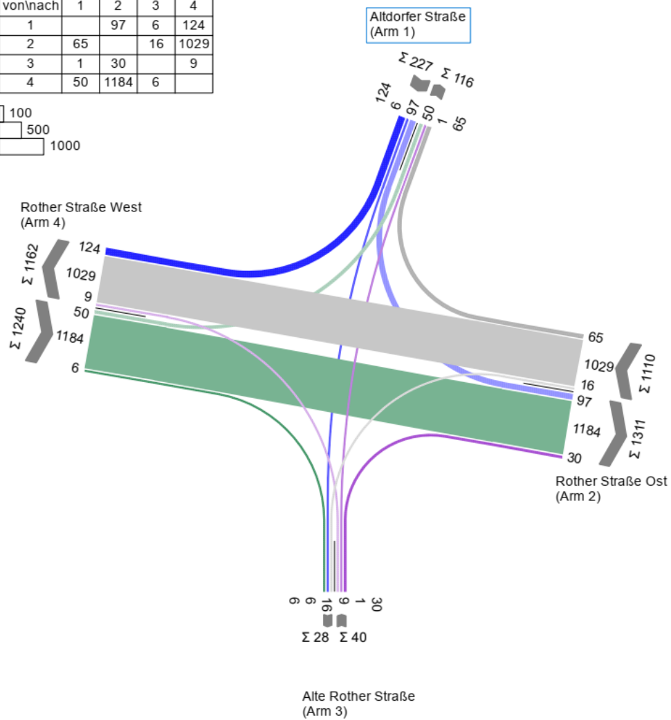
Anhang 93: KP 33 Strombelastungsplan Prognosenußfall 2030, Abendspitze
