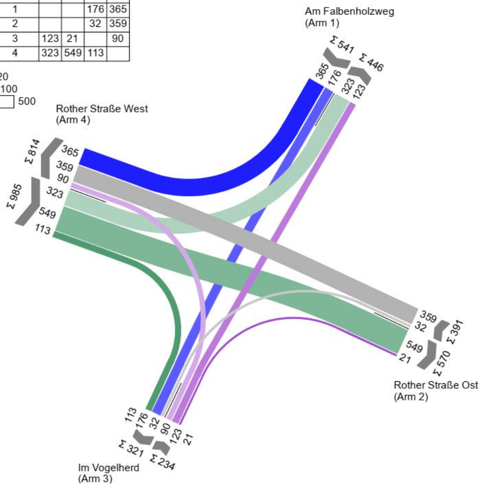
Anhang 33: KP 5 Strombelastungsplan Prognosenußfall 2030, Abendspitze
