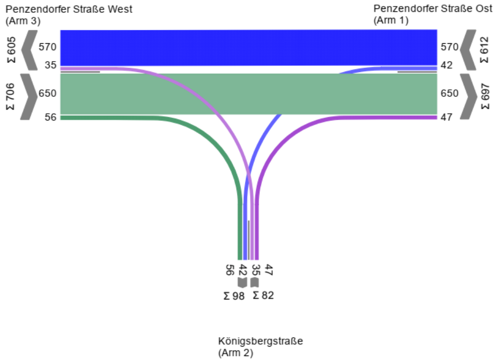
Anhang 129: KP 36 Strombelastungsplan Prognosenußfall 2030, Abendspitze
