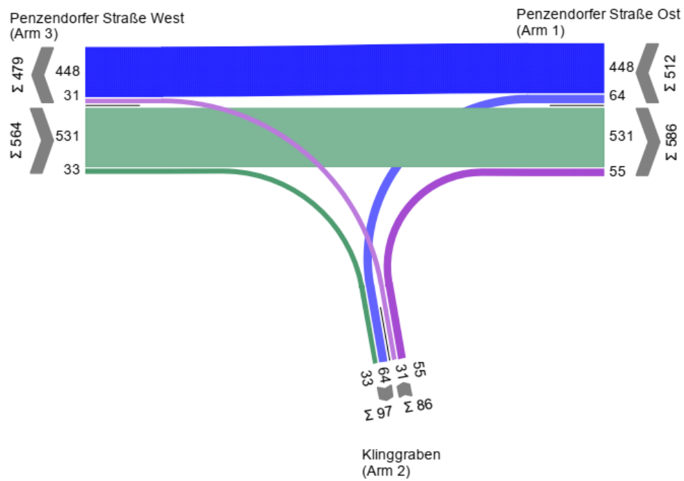
Anhang 105: KP 34 Strombelastungsplan Prognosenußfall 2030, Abendspitze
