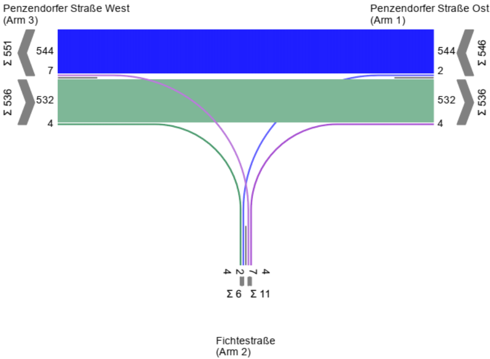
Anhang 141: KP 37 Strombelastungsplan Prognosenußfall 2030, Abendspitze
