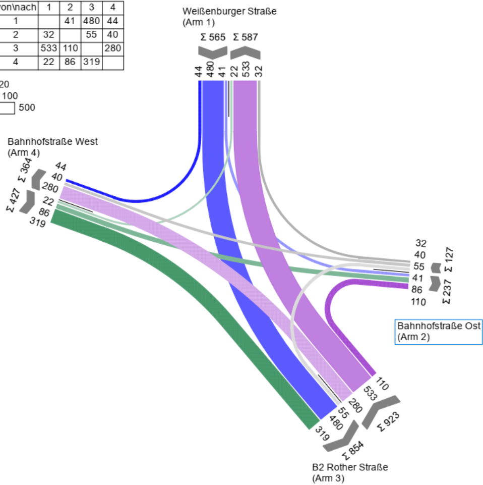
Anhang 8: KP 3 Strombelastungsplan Prognosenußfall 2030, Morgenspitze
