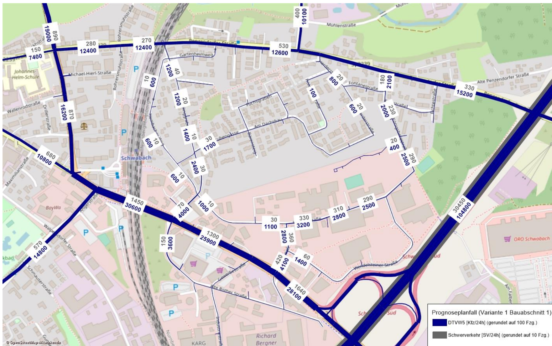
Abbildung 22: Umlegungsergebnis Variante 1.1, Bauabschnitt 1 (Kartengrundlage: Open Street Map)
