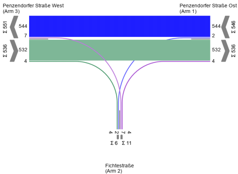
Anhang 140: KP 37 Strombelastungsplan Prognosenußfall 2030, Morgenspitze
