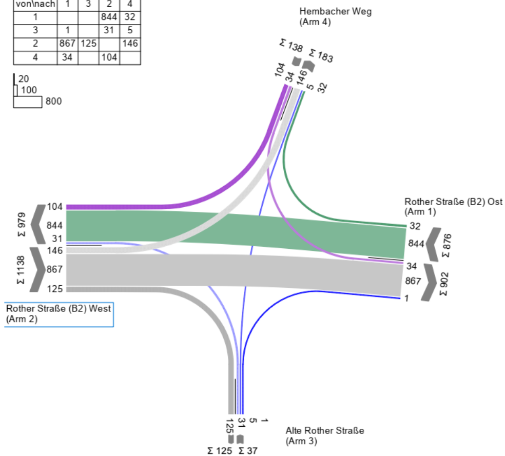
Anhang 84: KP 32 Strombelastungsplan Prognoseplanfall 2030, Morgenspitze
