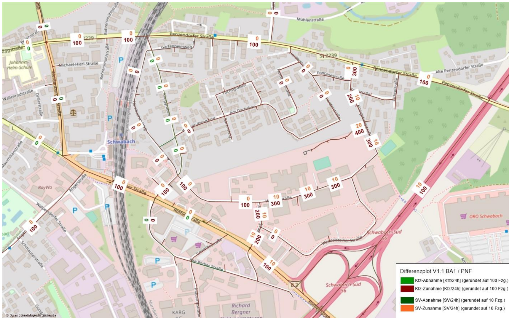
Abbildung 25: Differenzplot Variante 1.1, Bauabschnitt 1 + 2 / Prognosenullfall (Kartengrundlage: Open Street Map)
