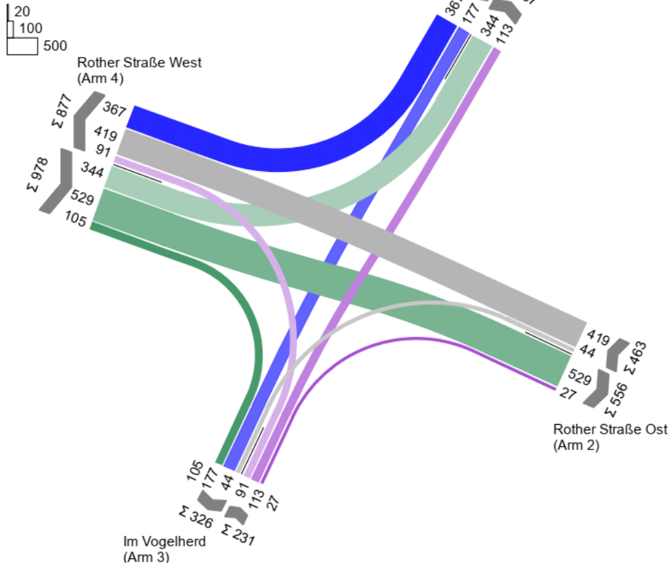
Anhang 29: KP 5 Strombelastungsplan Analyse 2018, Abendspitze
