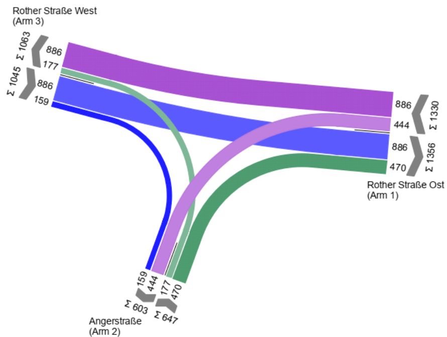
Anhang 21: KP 4 Strombelastungsplan Prognosenußfall 2030, Abendspitze
