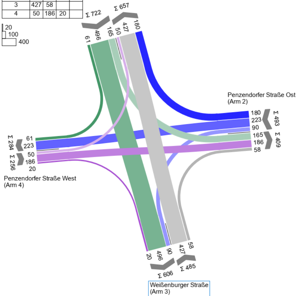
Anhang 44: KP 25 Strombelastungsplan Prognosenullfall 2030, Morgenspitze
