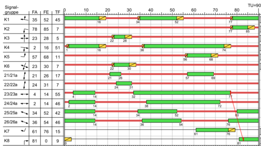
Abbildung 42: Signalzeitenplan des Knotenpunktes Rother Straße//Altdorfer Straße/alte Rother Straße (Quelle: LISA6.2.0)
