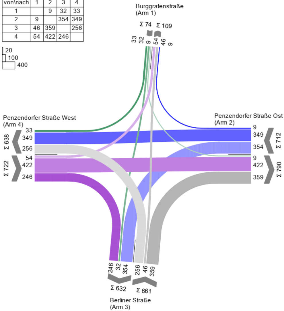
Anhang 56: KP 27 Strombelastungsplan Prognosenußfall 2030, Morgenspitze
