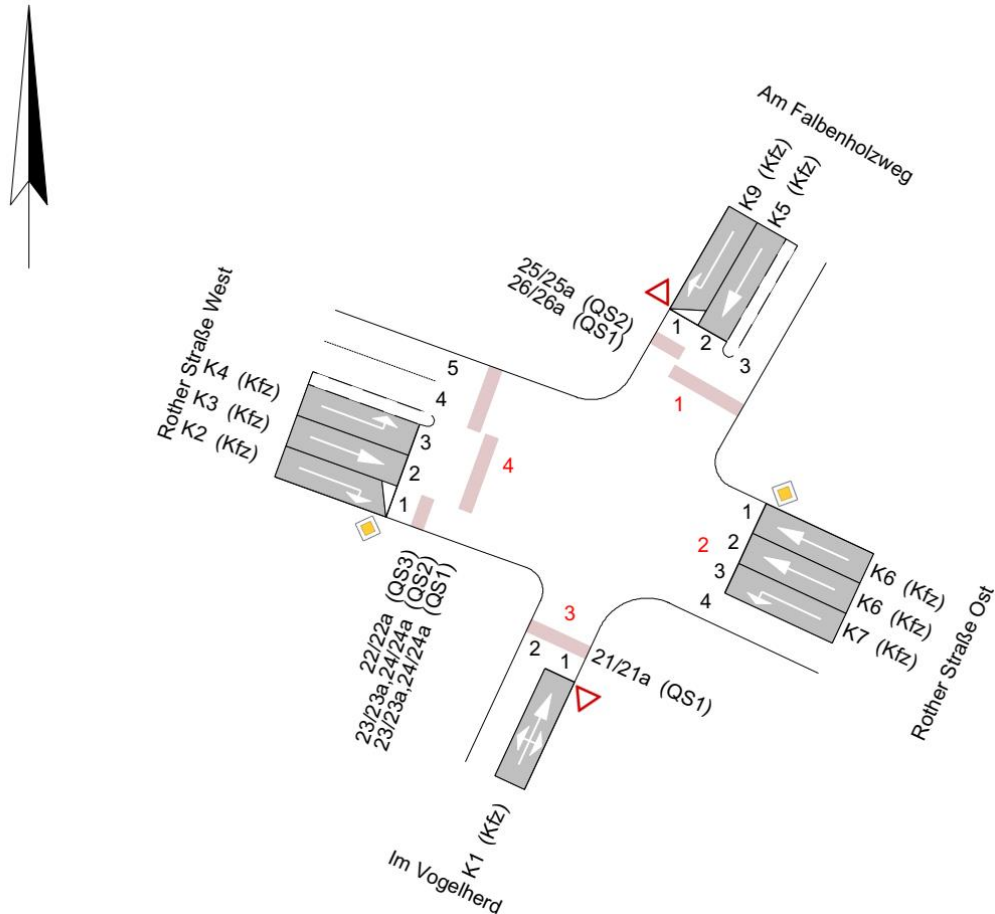
Abbildung 30: Geometrie des Knotenpunktes Rother Straße/Am Falbenholzweg mit Kennzeichnung der Nomenklatur (Quelle: LISA6.2.0)
