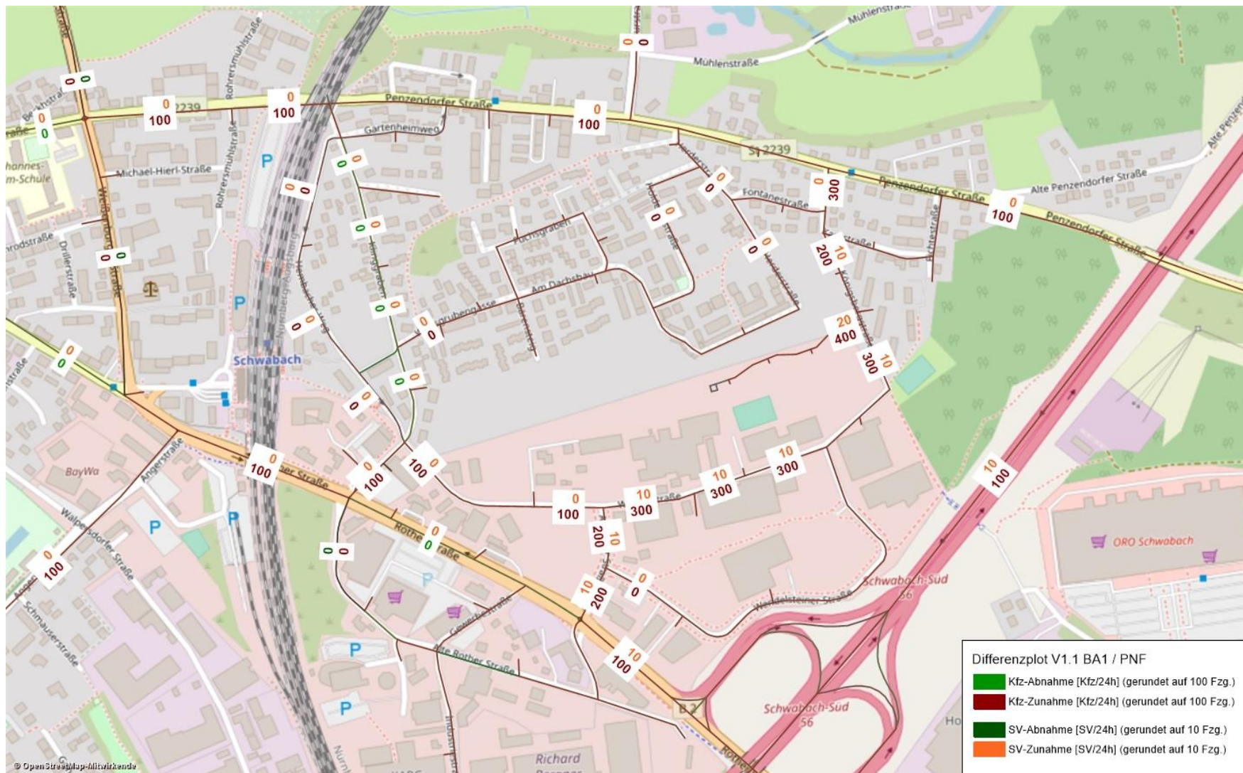
Abbildung 23: Differenzplot Variante 1.1, Bauabschnitt 1 / Prognosenußfall (Kartengrundlage: Open Street Map)
