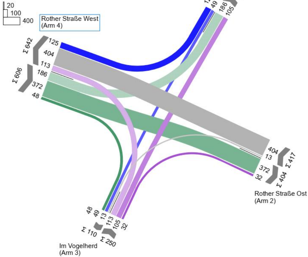
Anhang 32: KP 5 Strombelastungsplan Prognosenußfall 2030, Morgenspitze
