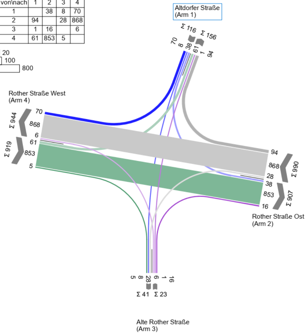
Anhang 92: KP 33 Strombelastungsplan Prognosenußfall 2030, Morgenspitze
