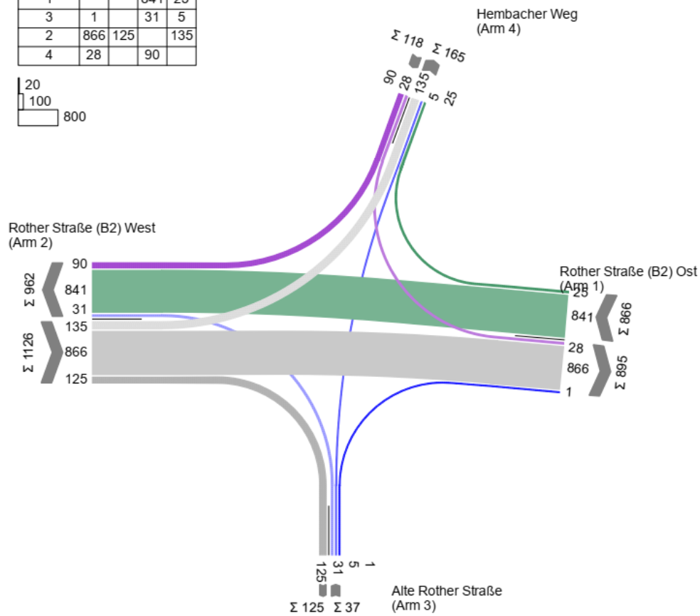
Anhang 80: KP 32 Strombelastungsplan Prognosenußfall 2030, Morgenspitze
