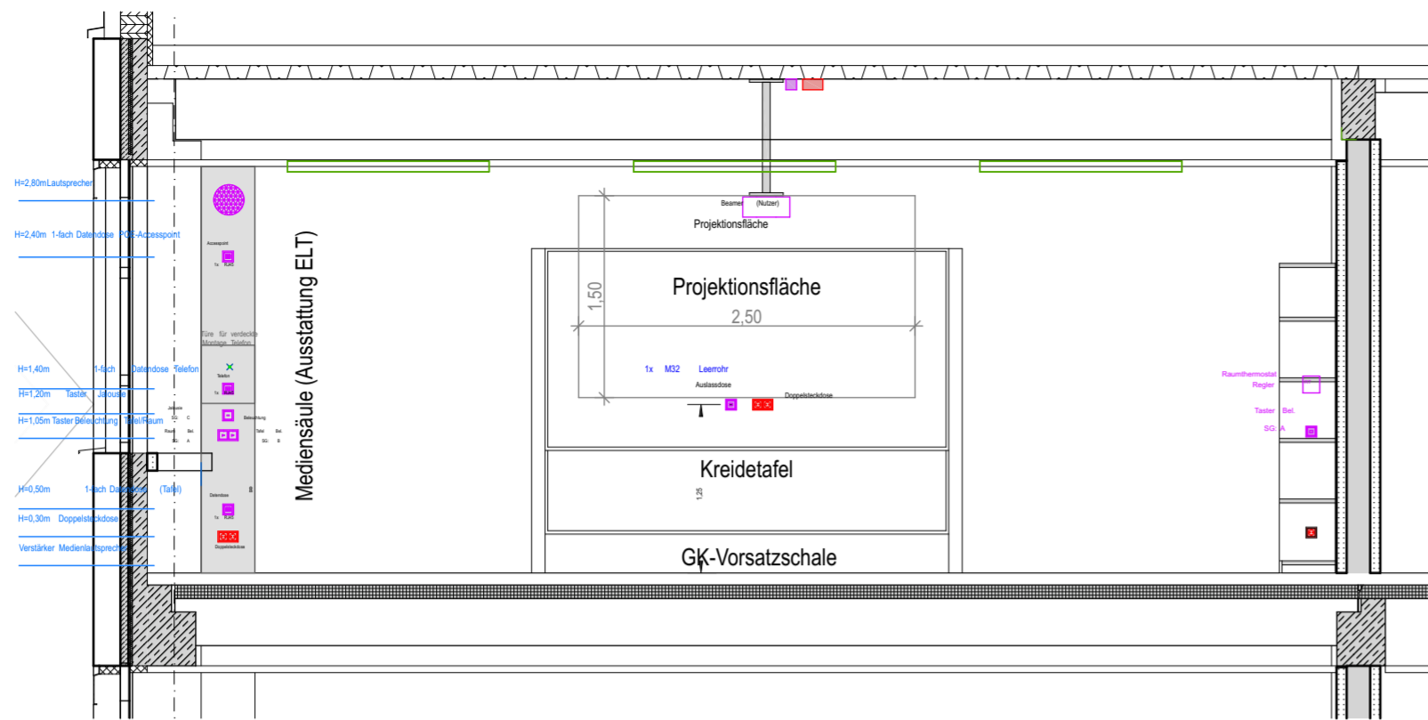
Ansicht Tafelwand
