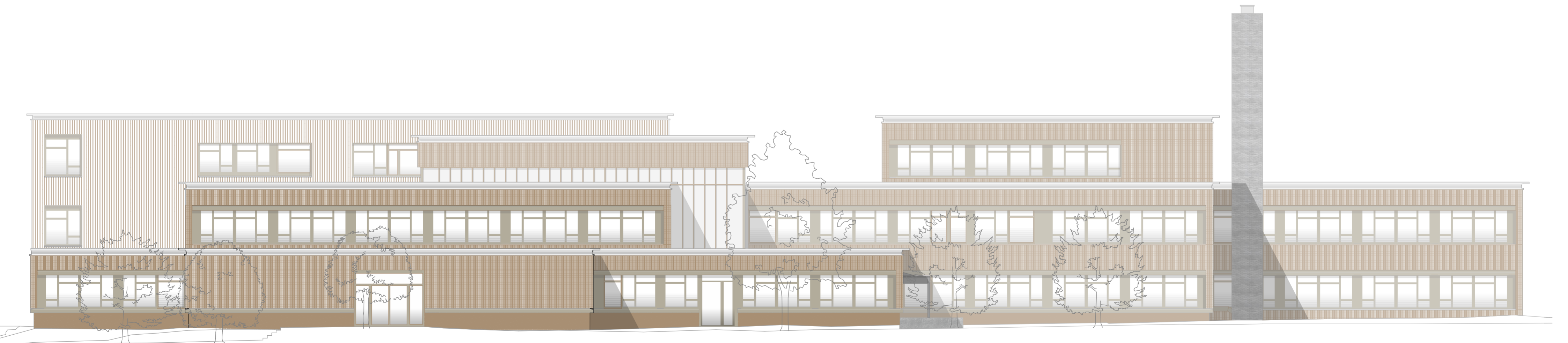
Ansicht Nord
