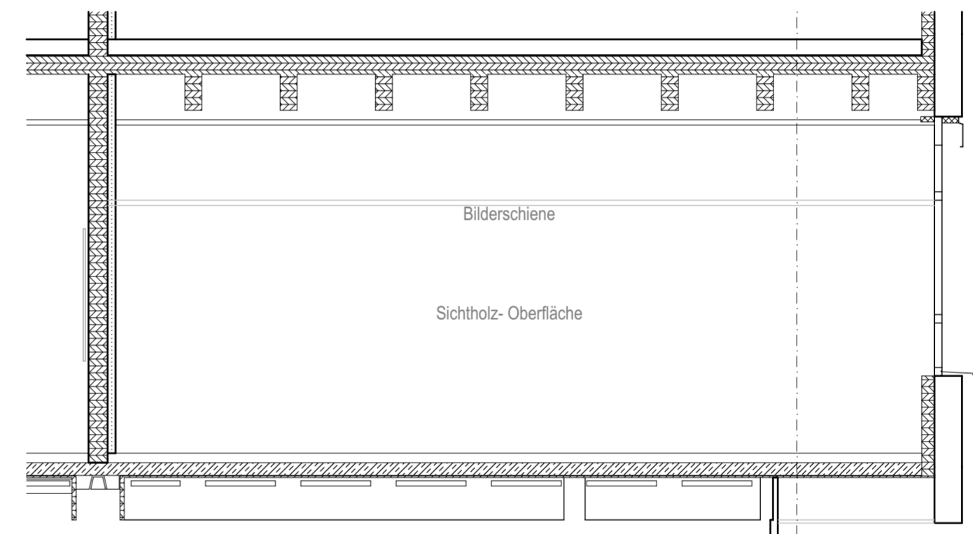
Ansicht Rückwand
