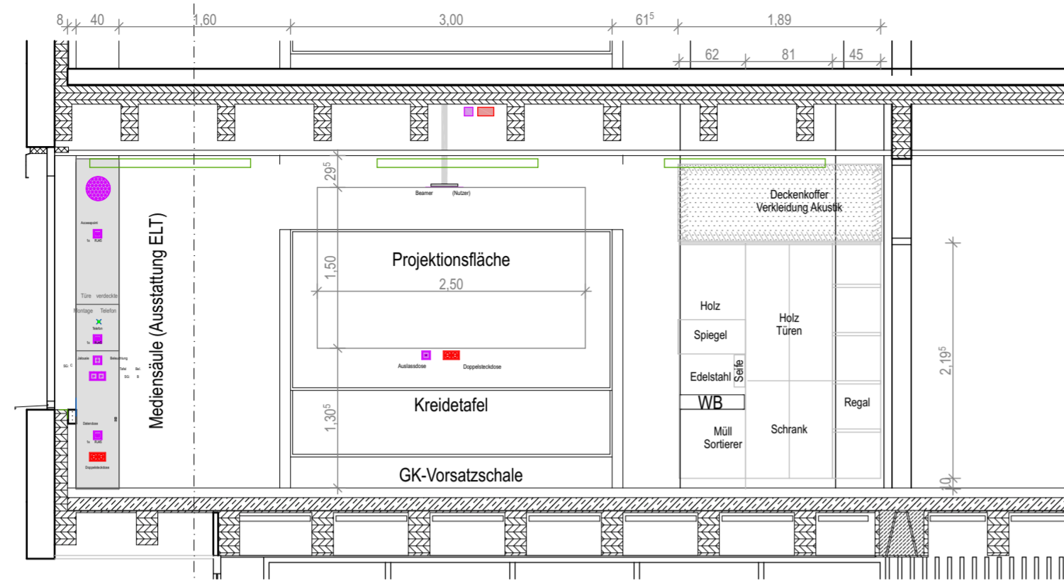
Ansicht Tafelwand
