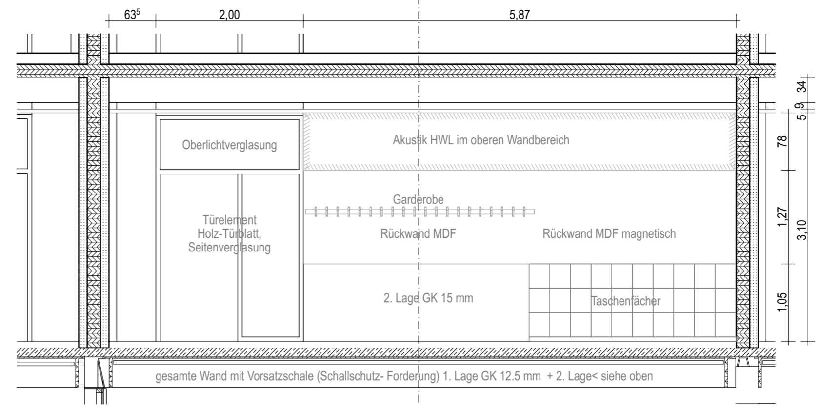
Ansicht Flurwand
