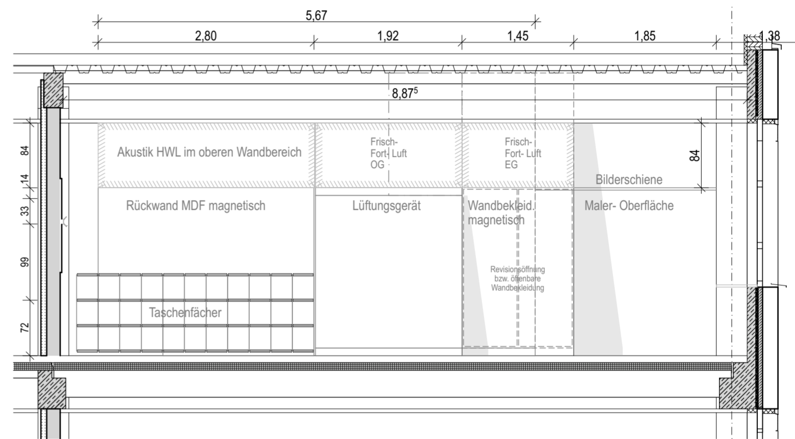
Ansicht Rückwand
