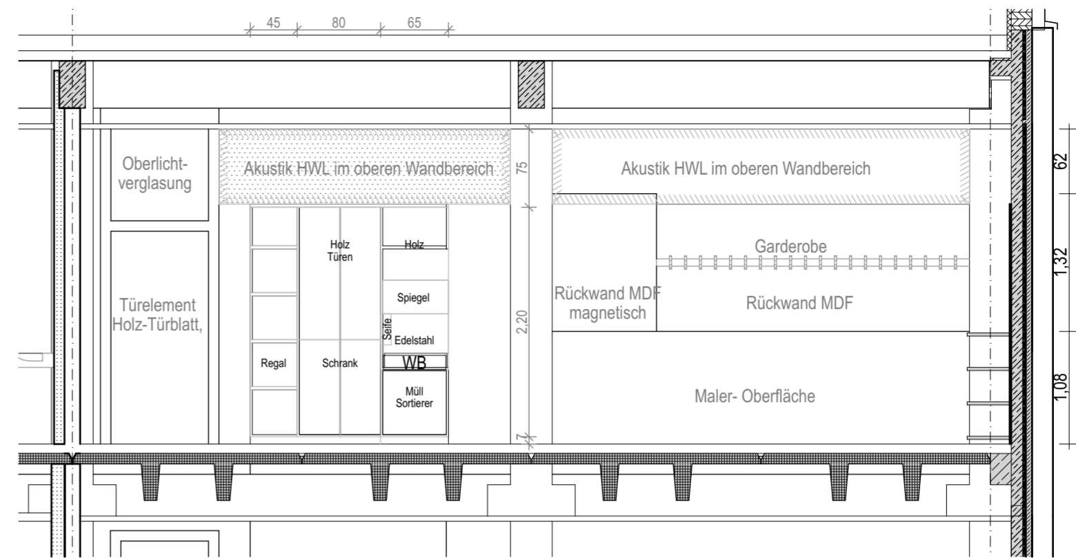
Ansicht Flurwand
