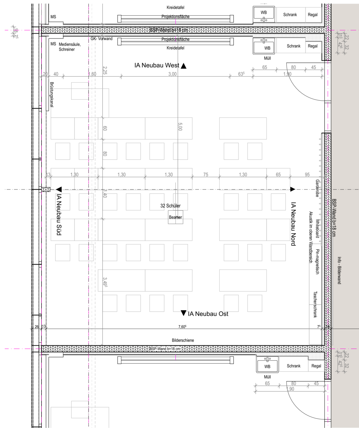
Grundriss
